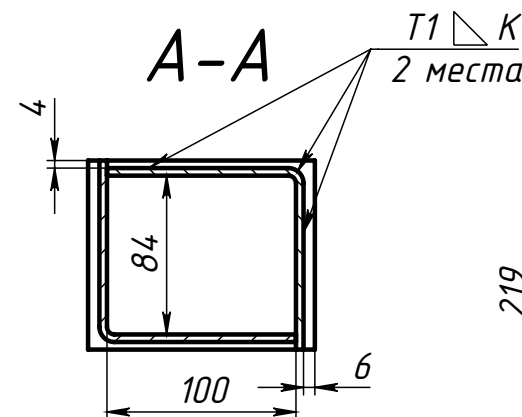
Поз.4 (Прокладка)
