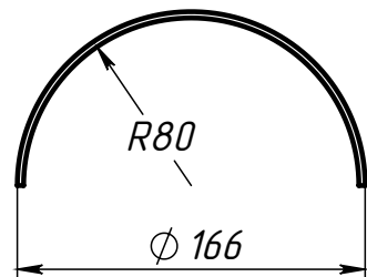
Поз.4 (Прокладка)
