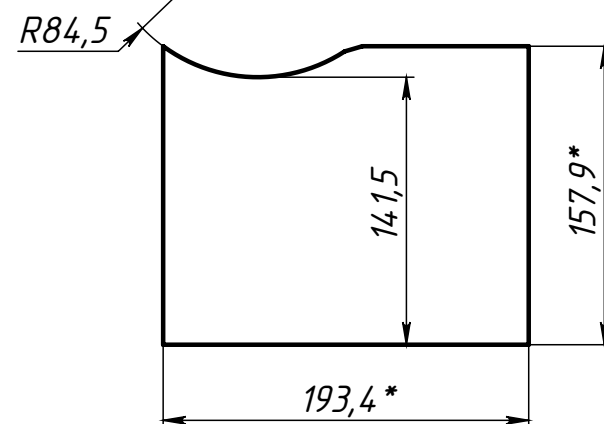
Поз.2 (Угольник) развертка
