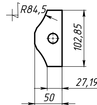
Поз.6 (Ушко) развертка
