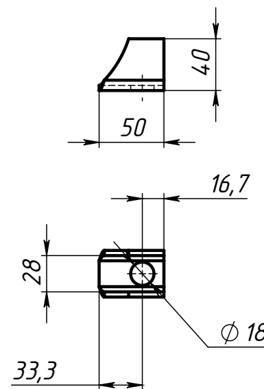
Поз.6 (Ушко)
